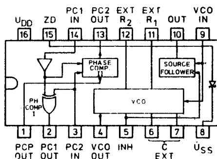
Układ wyprowadzeń
