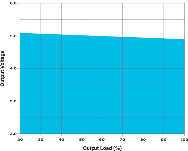
Output Load vs Output Voltage: MD112, Nom Line
