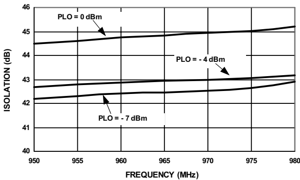
LO - IF Isolation vs. LO Power RF Power = -30 dBm
