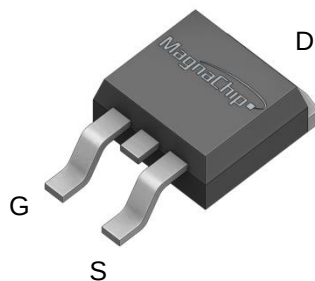
TO-263
