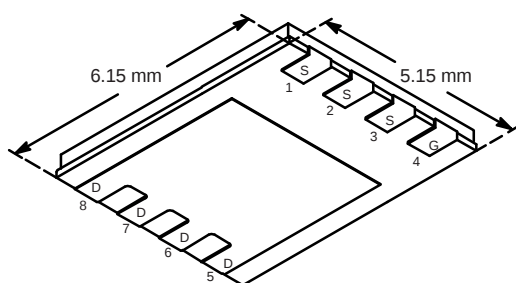
DFN8(5*6)
