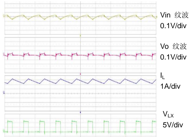
Fig.5 满载工作 2µs/div
