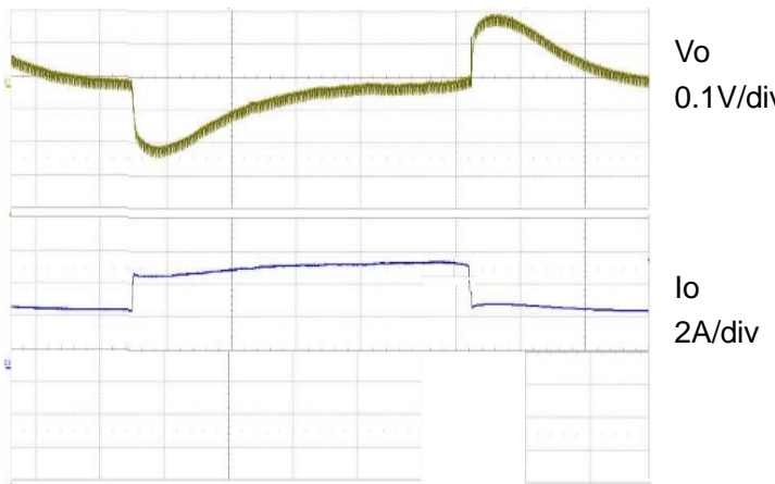
Fig.8 50% 到 100%负载瞬态 10µs/div
