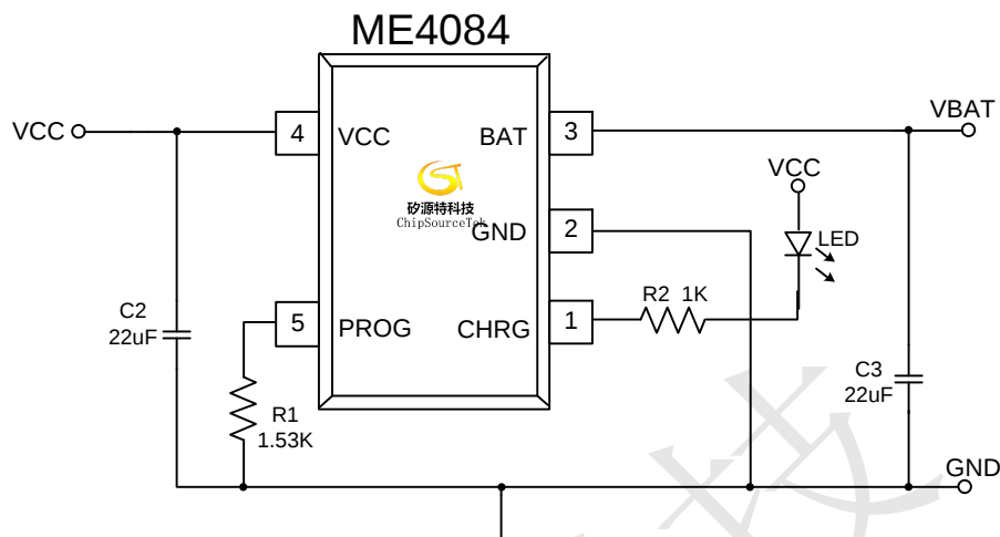
ME4084A典型应用原理图
