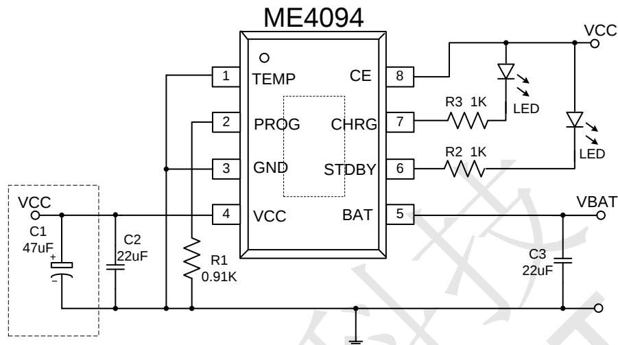
ME4094典型应用原理图
