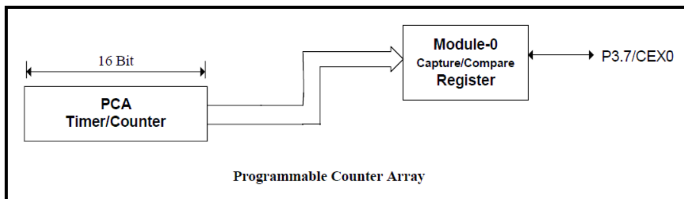
图13-1. PCA 方框图
