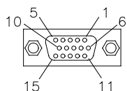
VGA
