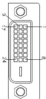
DVI-D
