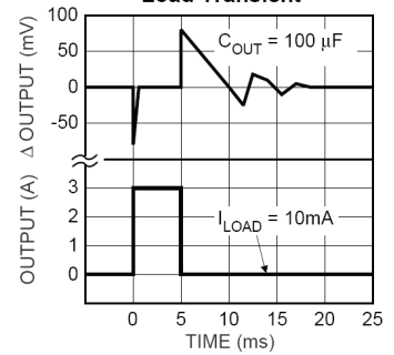
D2632 Load Transient
