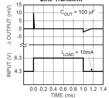
D2632 Line Transient
