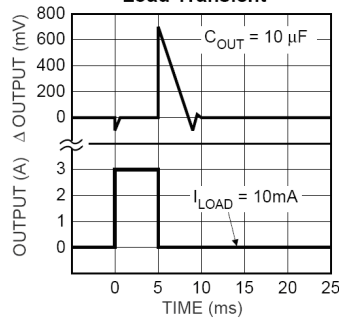
D2632 Load Transient
