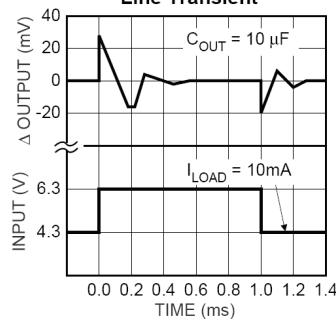
D2632 Line Transient
