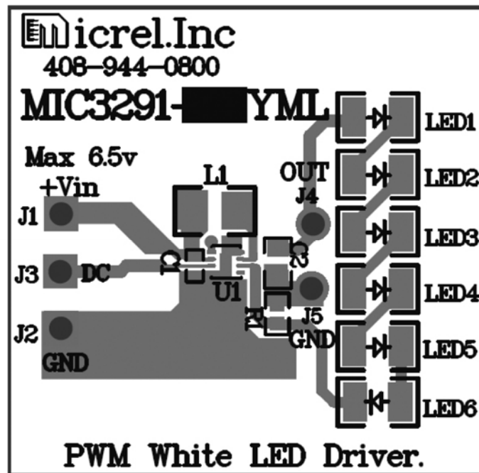
Top Layer
