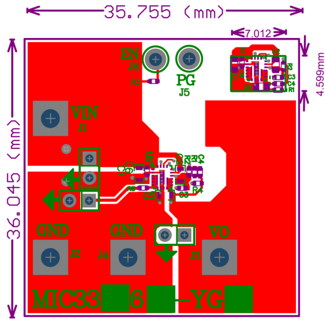
Top Layer
