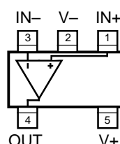
SOT-23-5 or SC-70
