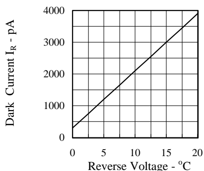
FIG.1 DARK CURRENT VS REVERSE VOLTAGE T AMB =25°C, E e =0 mW/cm 2
