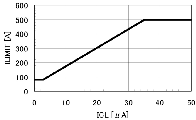
ILIMIT - ICL
