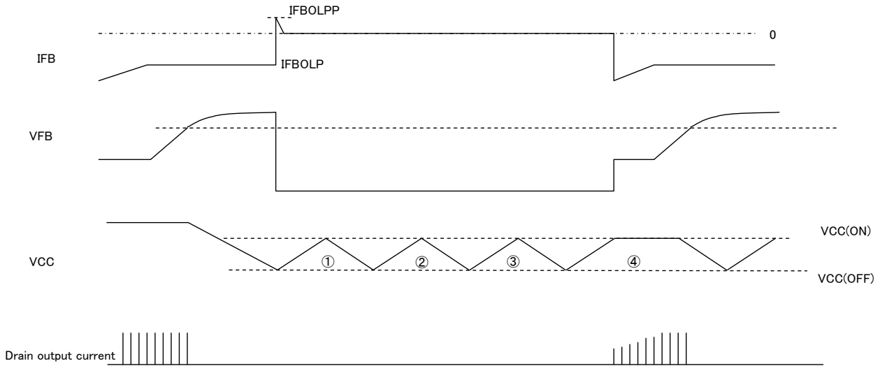
【Figure 3: Timer intermittent Over load protection diagram】
