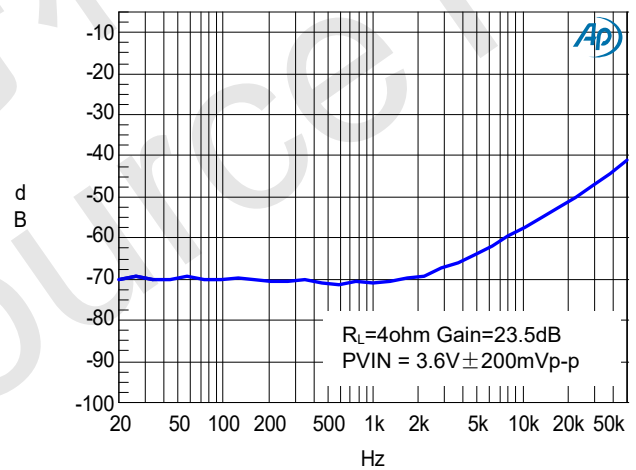
PSRR
