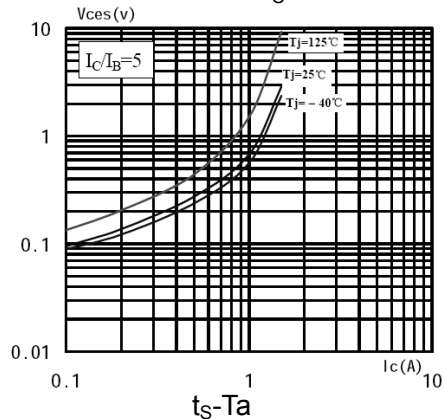
V_{CES}-I_C
