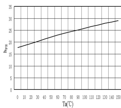
h FE -T a
