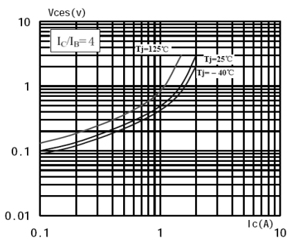
V ces -I C
