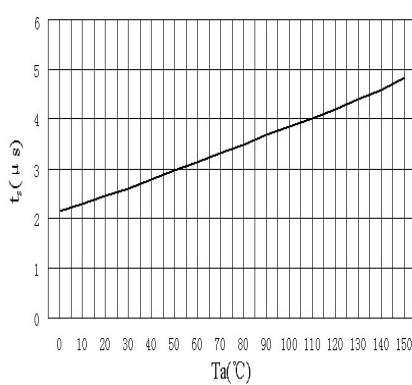
t S -T a
