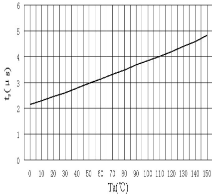
t_s - T_a
