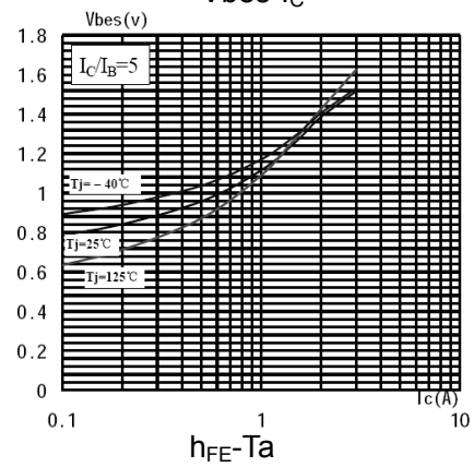
V_{bes}-I_C
