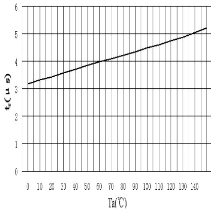
t_s-Ta
