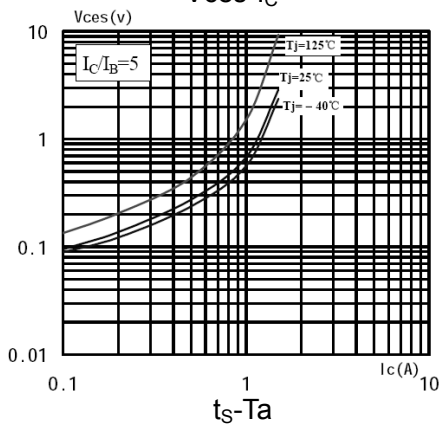
V_{ces}-I_C
