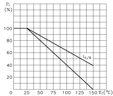
P_c - T_c
