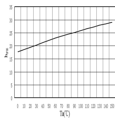
h_{FE}-T_a
