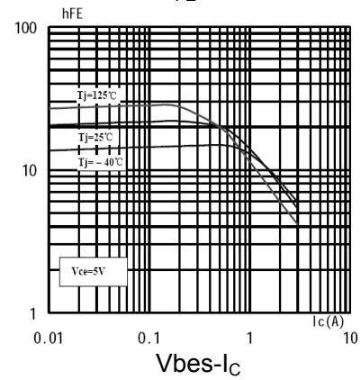
h_{FE}-I_C
