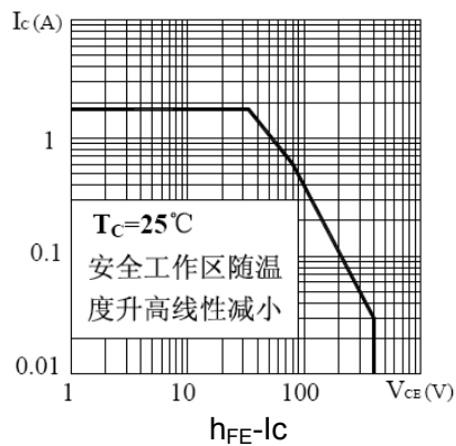
SOA(DC)
