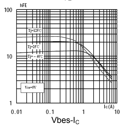
h_{FE}-I_C
