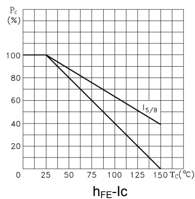
P_C-T_C
