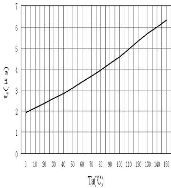
ts-Ta
