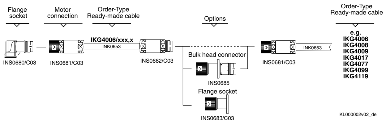
Fig. 17-2: Kabelauswahl INS0680 – 1,0mm 2
