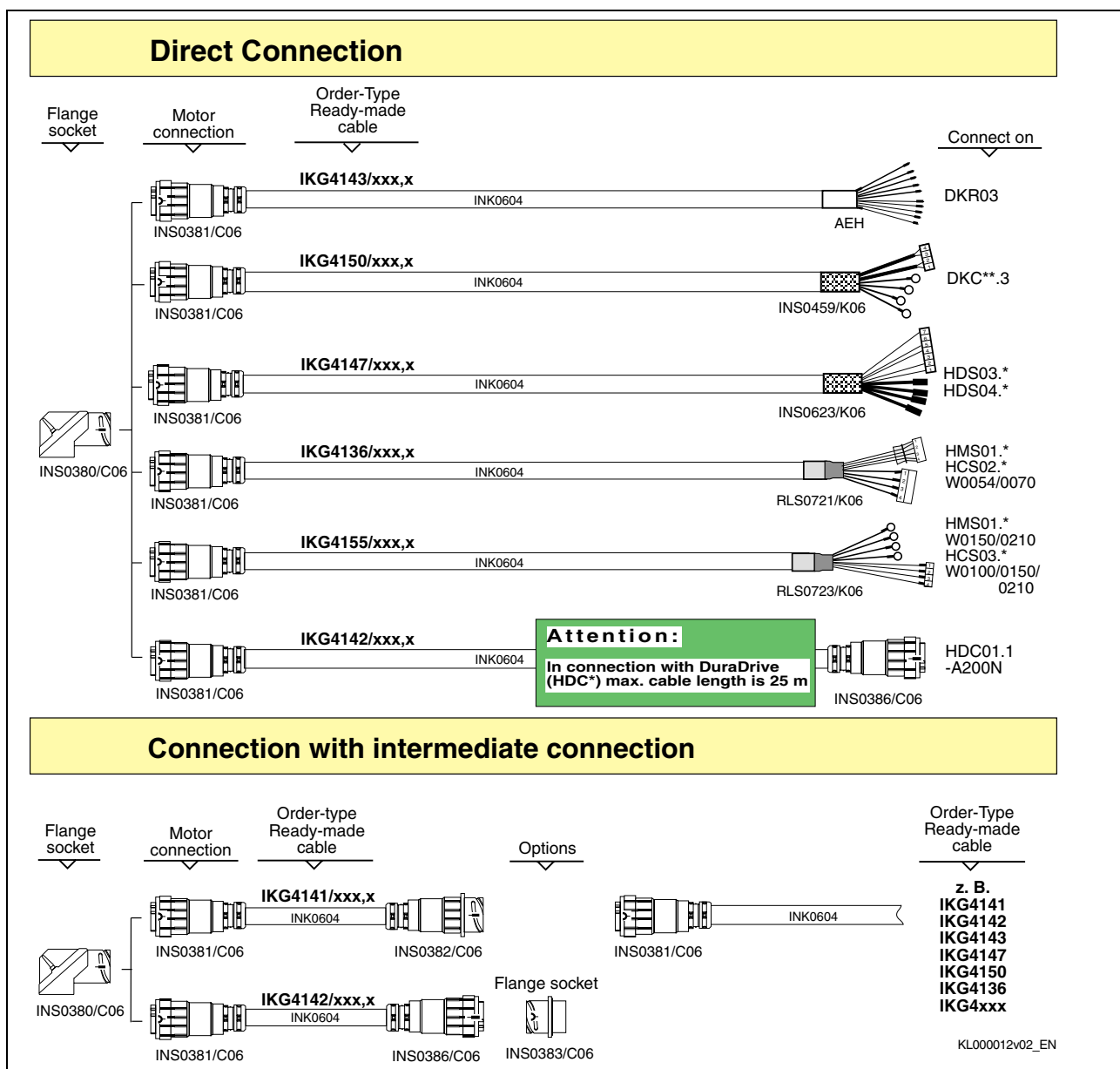
Fig. 17-9: Kabelauswahl INS0380 – 6,0mm 2
