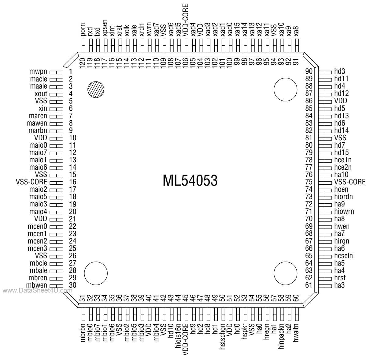
120-Pin Plastic TQFP
