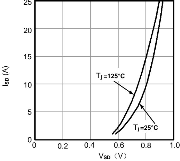
Figure4. Source-Drain Voltage
