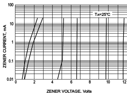
Zener Voltage Vs. Zener Current
