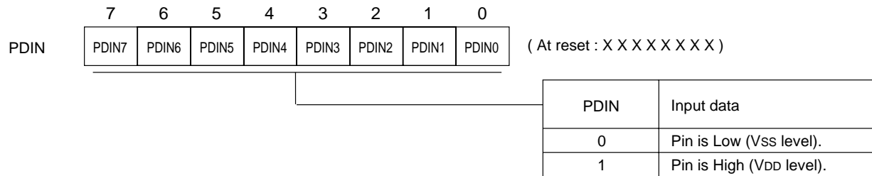
Port D input register (PDIN : x'03F2D', R)
