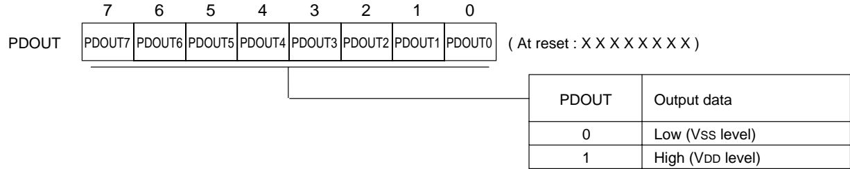
Port D output register (PDOUT : x'03F1D', R/W)
