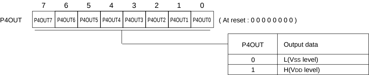
Port 4 output register (P4OUT : x'03F14', R/W)
