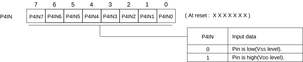
Port 4 input register (P4IN : x'03F24', R)
