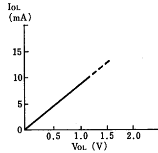
出力電流
