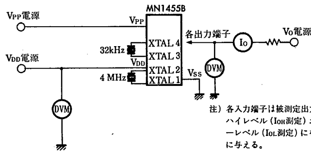
測定回路
