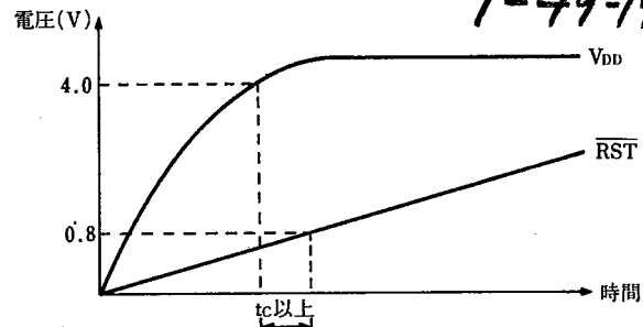
Fig. 5 イニシャルリセット回路および電圧波形
