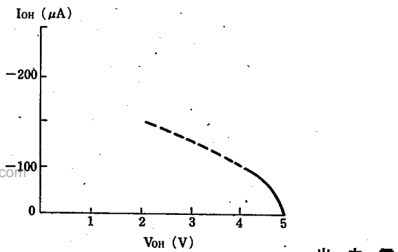
出力電流
