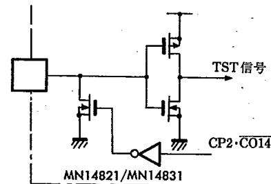
オープンドレイン出力回路(TST端子のみ)
