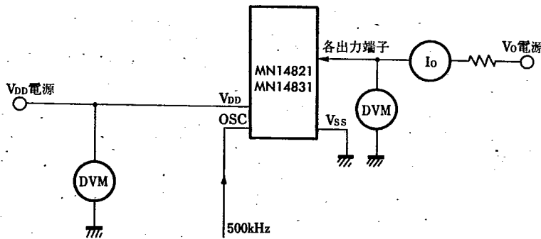
測定回路
