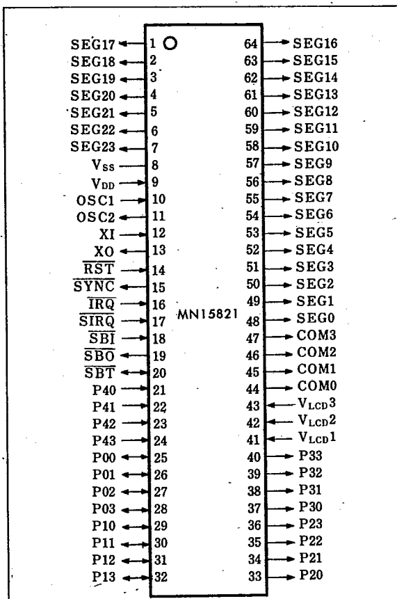
Ⓞ 64-SDIP
