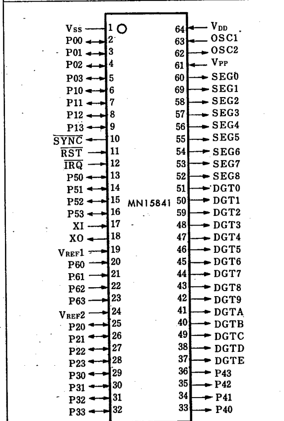
Ⓞ 64-SDIP
