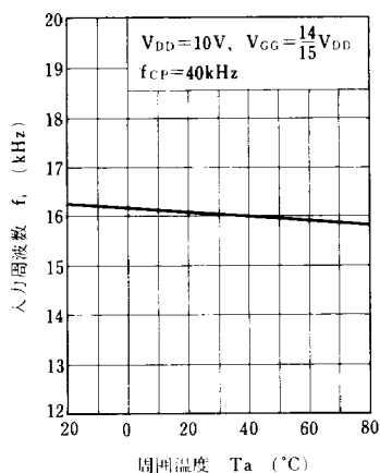
f_i - T_a
