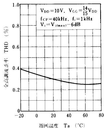
THD - T_a
