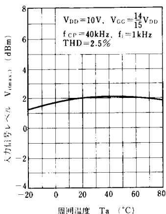
V_{i(max)} - T_a
