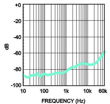
PSRR Test
