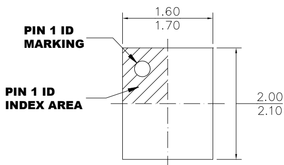
WLCSP20 (1.6mmx2.0mm)
