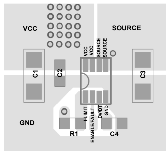
Top Layer
