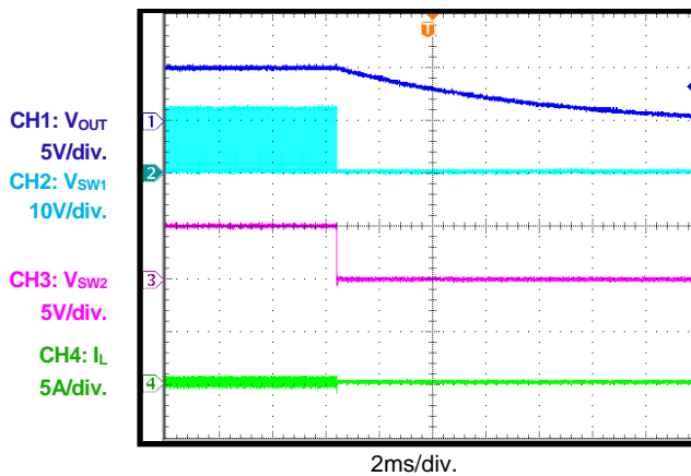
EN Pin Disable Load = 0A
