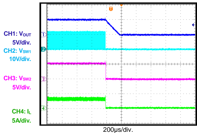
EN Pin Disable Load = 3A
