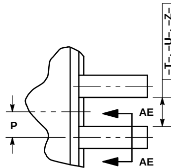
DETAIL Y
