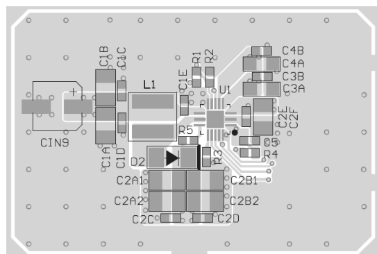
Top Layer
