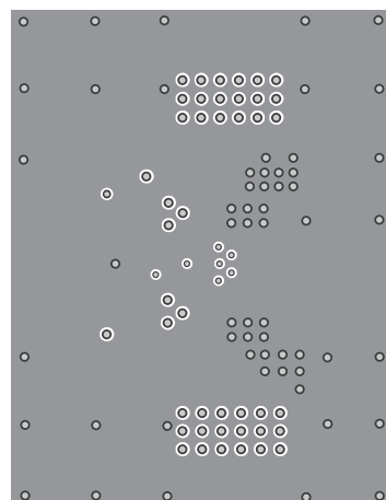
Bottom Layer
