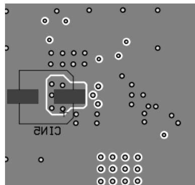
Bottom Layer
