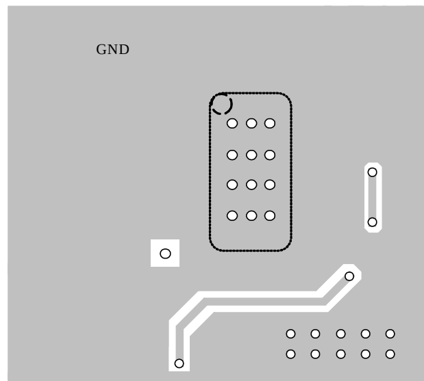
Bottom Layer
