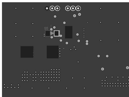
Bottom Layer
