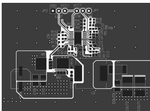
Top Layer
