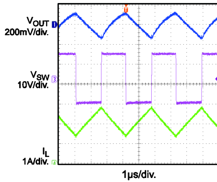
VOUT Ripple
