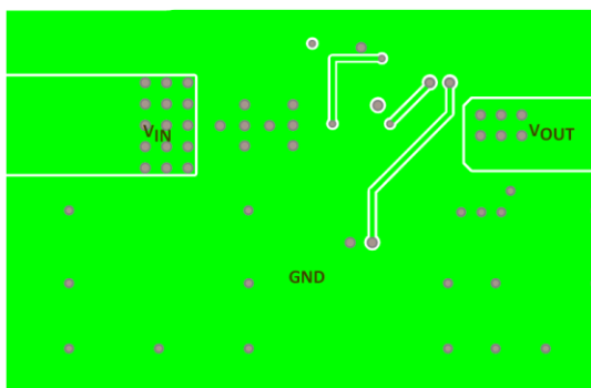
Inner Layer 2
