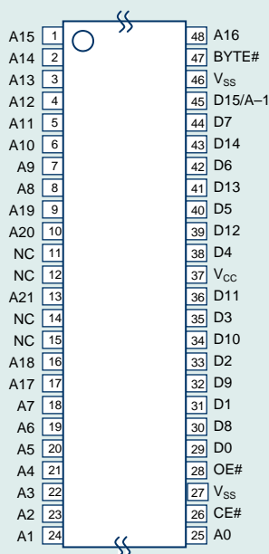
48TSOP(Type-I)
