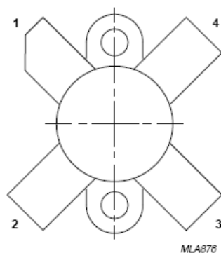
SOT121
